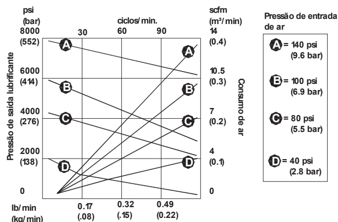
Gráfico de desempenho P-225/50
