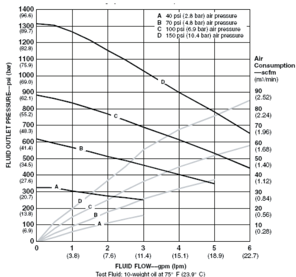
Gráfico de desempenho P-425/10
