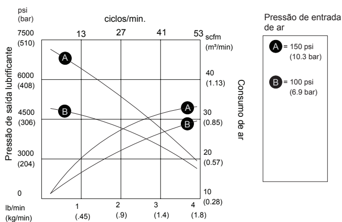
Gráfico de desempenho P-425/50
